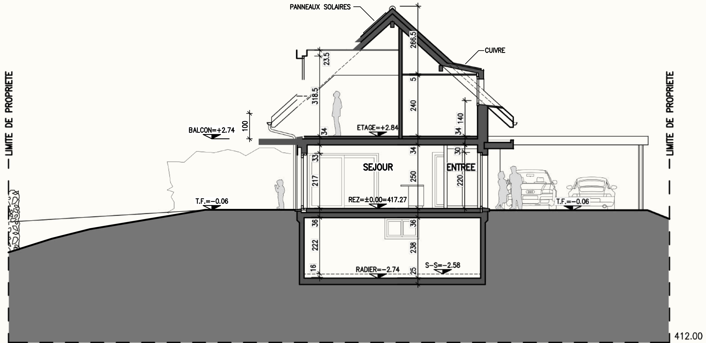
COUPE A-A
