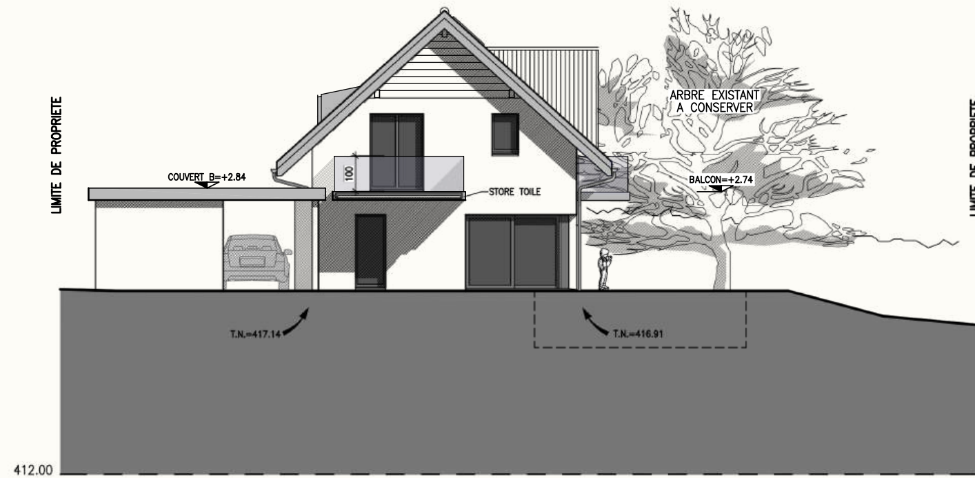
FAÇADE SUD-OUEST
