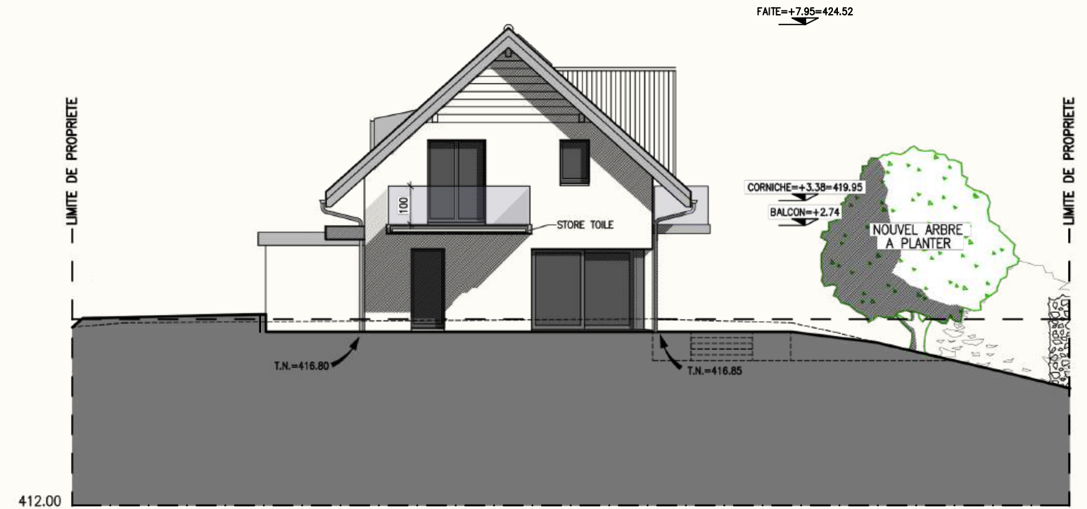
FAÇADE SUD-OUEST
