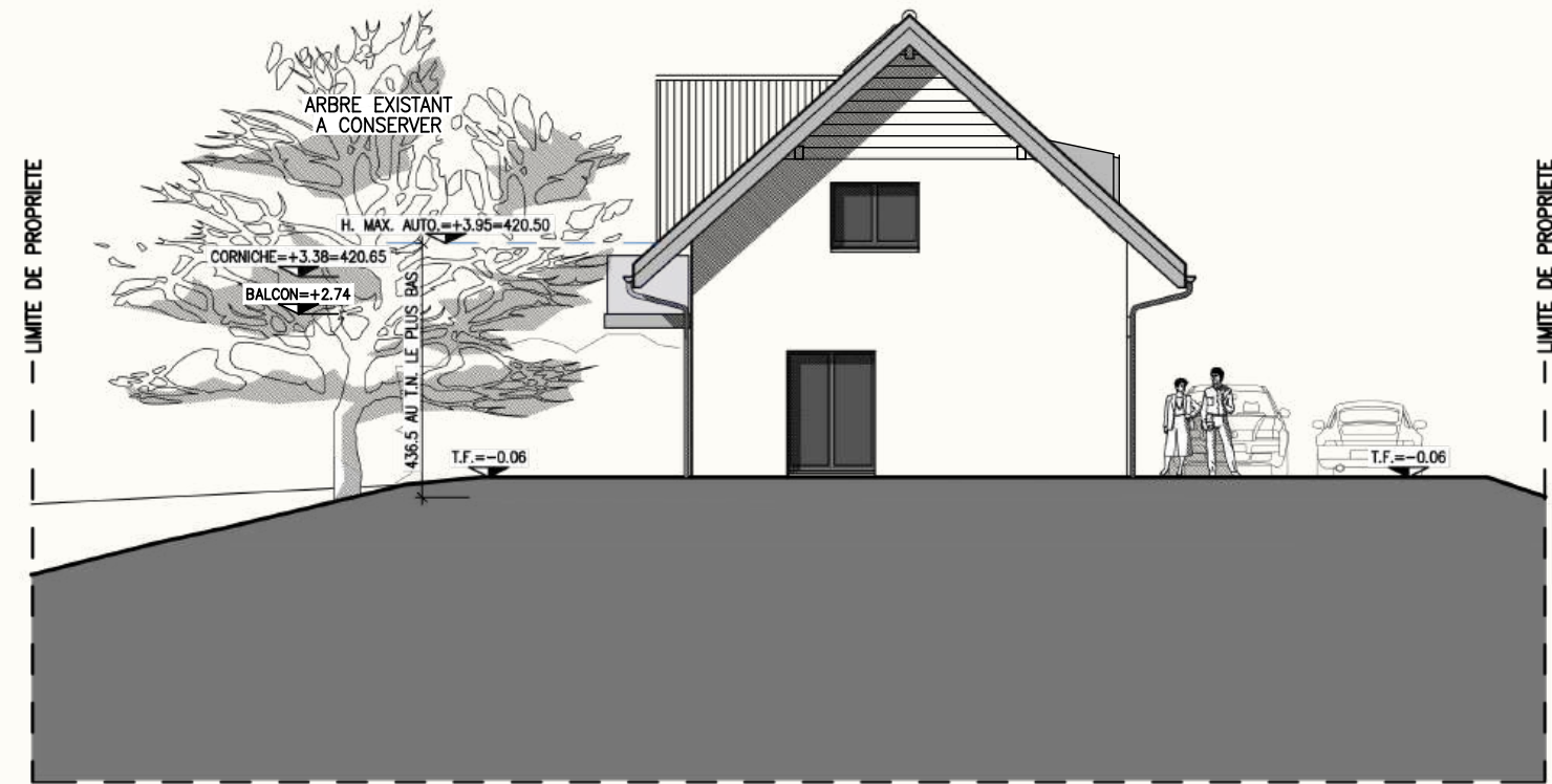
FAÇADE NORD-EST
